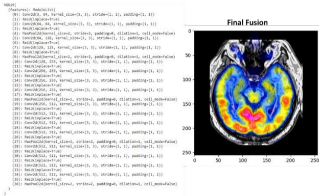
Fig. 7. VGG19 Fusion
